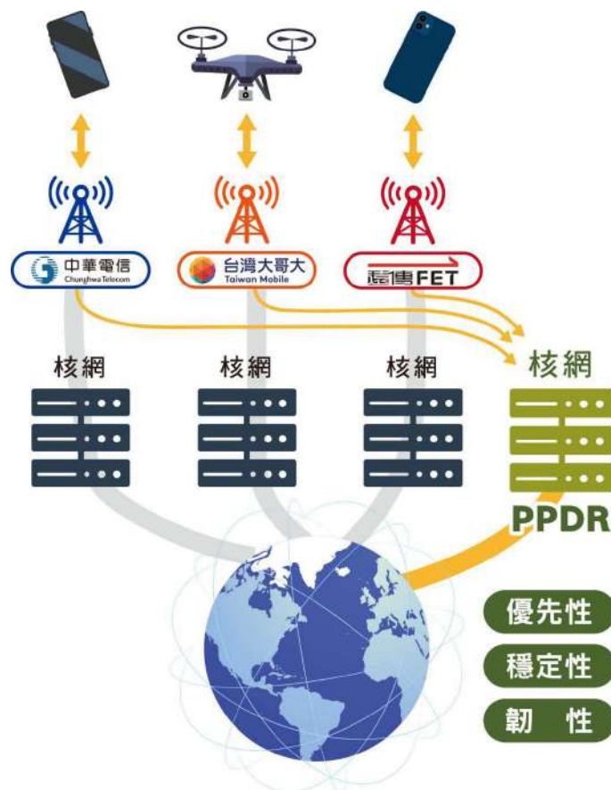
圖 3-22、113 年概念性驗證多營運商核心網路（Multi-Operator Core Network, MOCN）技術示意圖
